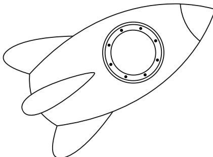
ESPAZIO-ONTZI
