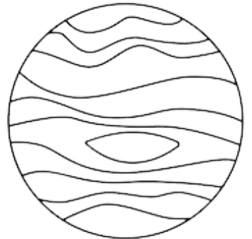
JUPITER
