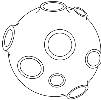
MARTE
