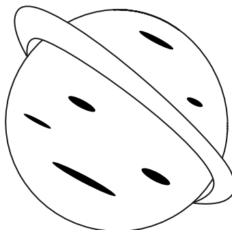
URANO
