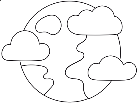
LURRA
