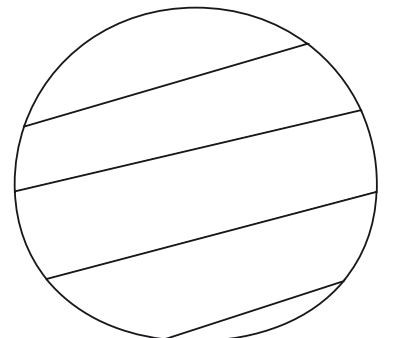
NEPTUNO
