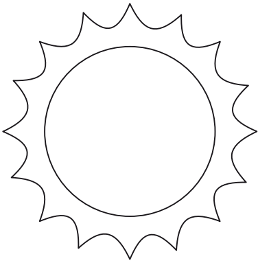
EGUZKIA
