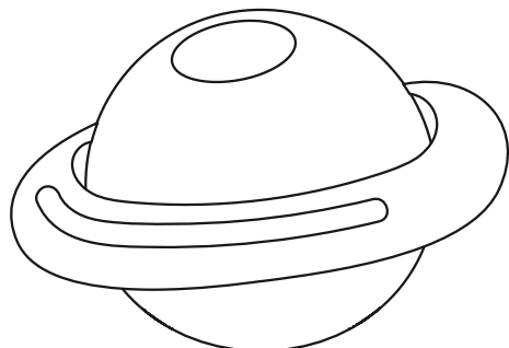
SATURNO
