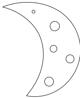
ILARGIA
