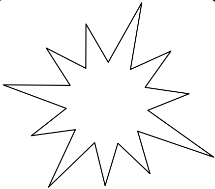
IZARRA
