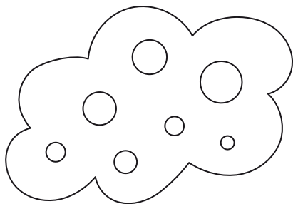
NEBULOSA
