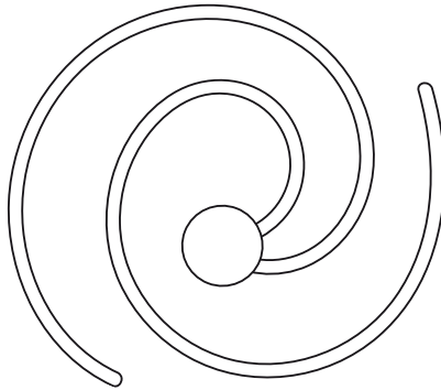
GALAXIA
