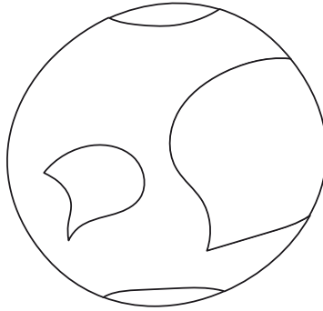
MERKURIO
