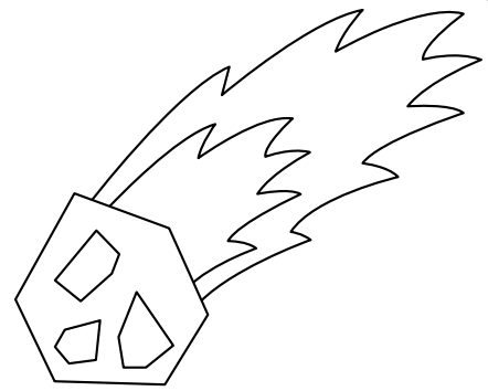
METEORITOA
